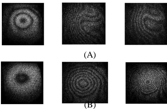
Gambar 3. (A) Perubahan bentuk pola frinji karena perubahan frekuensi; (B) Perubahan jumlah frinji karena perubahan amplitudo.
