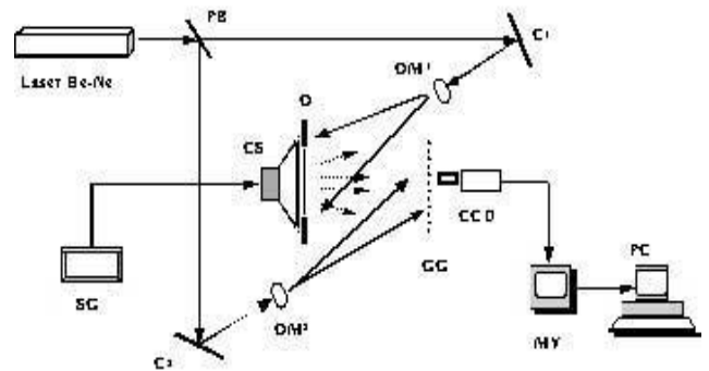
Gambar 2. Skematik susunan komponen percobaan
