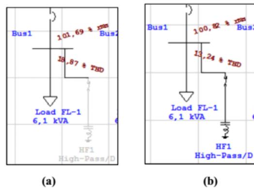
Gambar 5. a. Tampilan THDi pada beban FL-1 sebelum pemasangan filter; b. Tampilan THDi pada beban FL-1 setelah pemasangan filter
