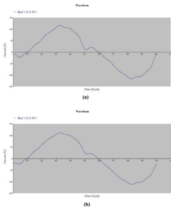
Gambar 7. a. Bentuk gelombang THDi FL-1 sebelum pemasangan filter; b. Bentuk gelombang THDi FL-1 setelah pemasangan filter
