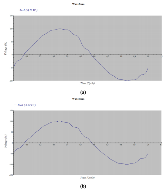
Gambar 6. a. Bentuk gelombang THDv FL-1 sebelum pemasangan filter; b. Bentuk gelombang THDv FL-1 setelah pemasangan filter
