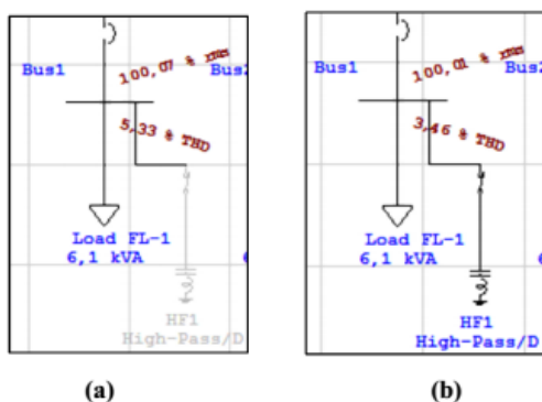
Gambar 4. a. Tampilan THDv pada beban FL-1 sebelum pemasangan filter; b. Tampilan THDv pada beban FL-1 setelah pemasangan filter
