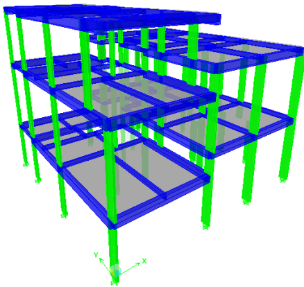
Gambar 5. Pemodelan 3 dimensi
