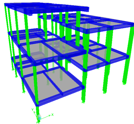
Gambar 2. Pemodelan 3 dimensi
