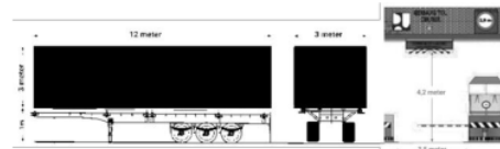
Gambar 6: Dimensi Modul Volumetrik Maksimal Sumber: Analisis, (2023)
