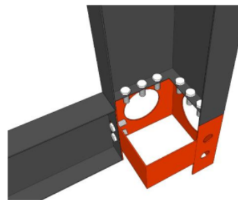
Gambar 16: Sambungan Modul Sumber: Analisis, (2023)
