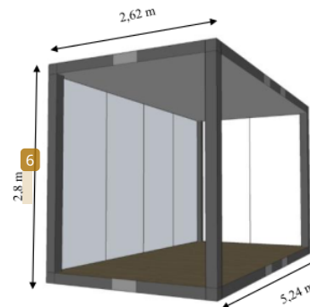
Gambar 15: Struktur Rangka Utama Modul Sumber: Analisis, (2023)
