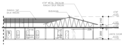
Gambar 7: Grid Vertikal Modul Rumah Sakit Pusat Pertamina Simprug Sumber: Analisis, (2023)
