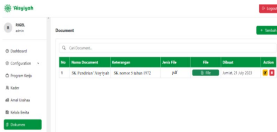
Gambar 9. Pengarsipan Dokumen
