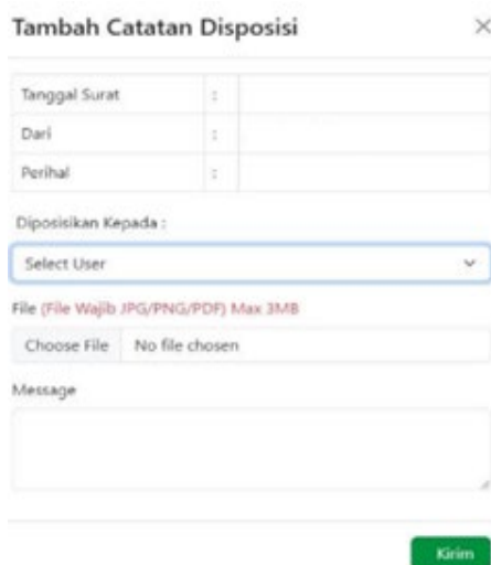
Gambar 6. Disposisi E-Surat
