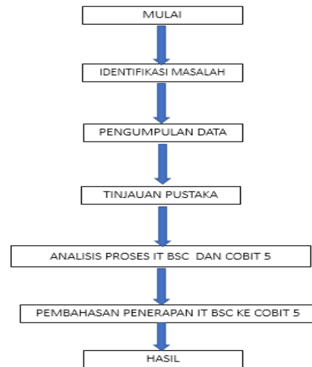
Gambar 1.2 Tahapan Penelitian
