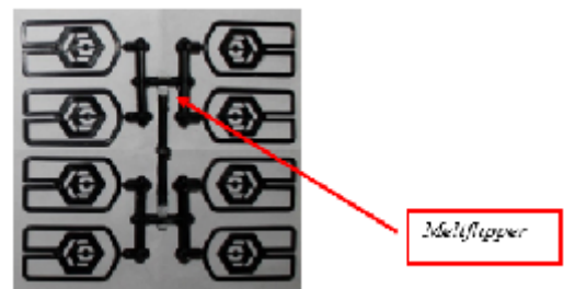
Gambar 17. Foto hasil trial Ke-2 (tanpa meltflipper ) dari Shot 27.
