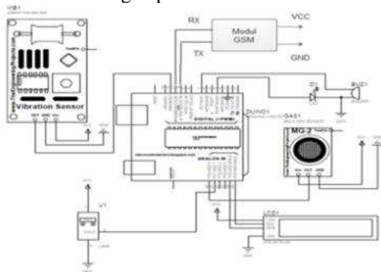
Gambar 12. Rangkaian sistem keseluruhan
