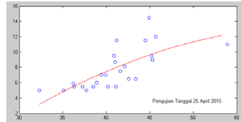
Gambar 4.3 Grafik hubungan antara temperatur dengan arus – 25 April 2015 Kurva diatas memiliki fungsi polynomial yaitu f(x) = -0,0049x^2 + 0,6574x - 11,9053 dengan error Rata-rata = 1,1004 atau 13,7%.
