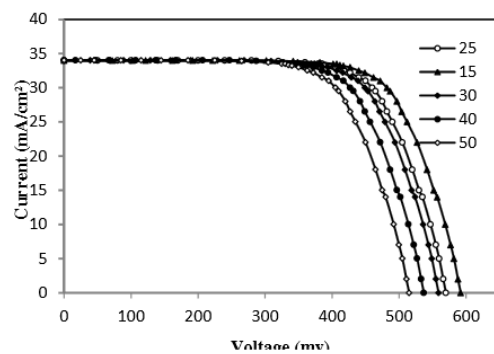
Gambar 2.6 Efek temperature pada karakteristik IV sel surya [2]
