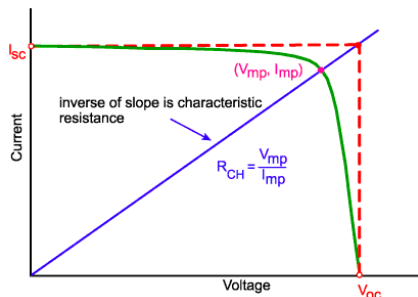
Gambar 2.4 Karakteristik resistansi [2]
