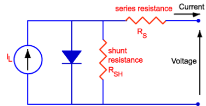
Gambar 2.5 Resistansi seri dan shunt pada rangkaian sel surya. [2]
