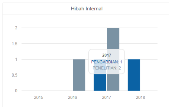
Gambar 12. Pola Grafik (2)
