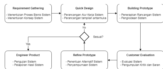
Gambar 1. Metode Prototipe
