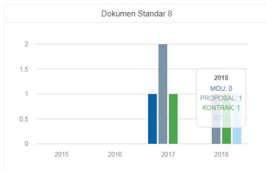
Gambar 11. Pola Grafik (1)
