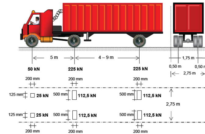
Gambar 3 Pembebanan Truk "T"
