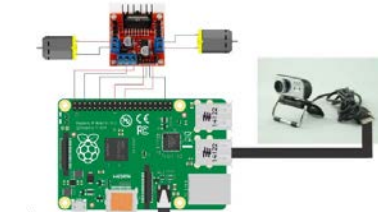
Gambar 4. Rangkaian Komponen
