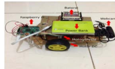
Gambar 5. Implementasi Robot
