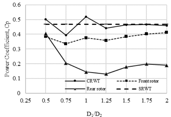
Gambar 14. Perbandingan koefisien daya turbin di setiap variasi rasio diameter pada TSR = 6
