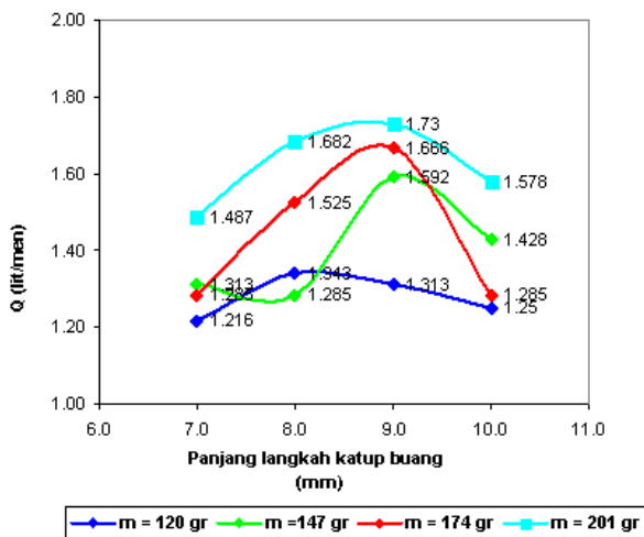
Gambar 9. Grafik hubungan panjang langkah katup buang terhadap debit pemompaan dan berat katup buang pada head pemompaan 8 m
