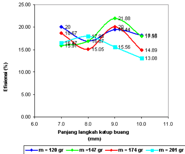
Gambar 12. Grafik hubungan panjang langkah katup buang terhadap efisiensi dan berat katup buang pada head pemompaan 9 m.
