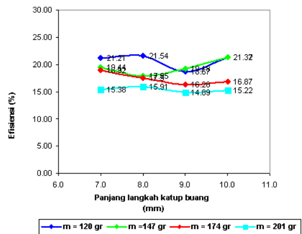
Gambar 10. Grafik hubungan panjang langkah katup buang terhadap efisiensi dan berat katup buang pada head pemompaan 8 m.
