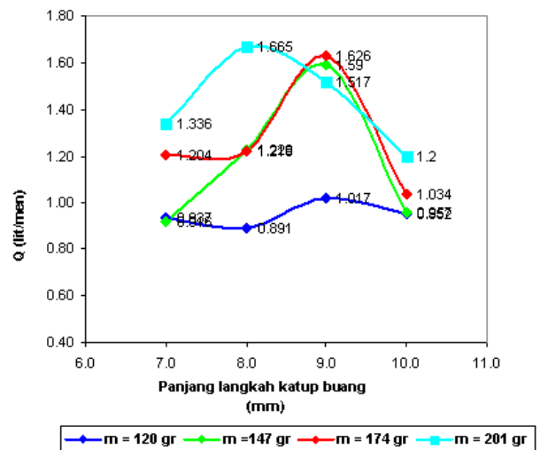
Gambar 11. Grafik hubungan panjang langkah katup buang terhadap debit pemompaan dan berat katup buang pada head pemompaan 9 m.
