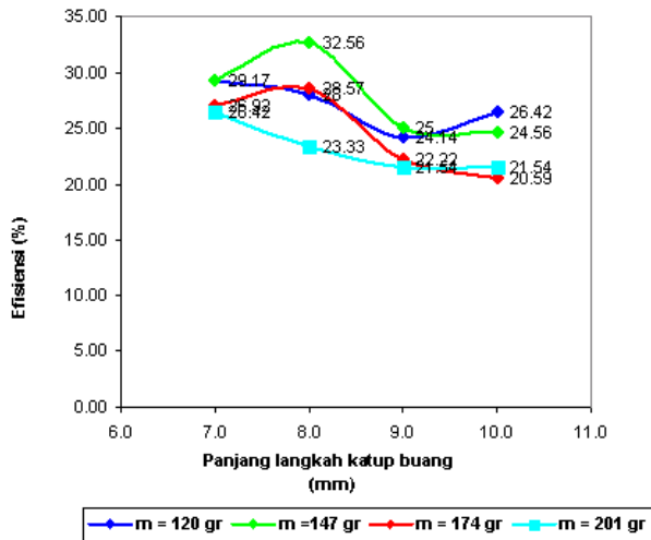
Gambar 8. Grafik hubungan panjang langkah katup buang terhadap efisiensi dan berat katup buang pada head pemompaan 7 m.
