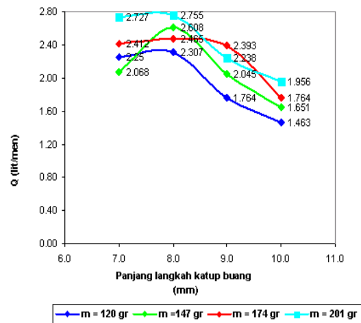
Gambar 7. Grafik hubungan panjang langkah katup buang terhadap debit pemompaan dan berat katup buang pada head pemompaan 7 m
