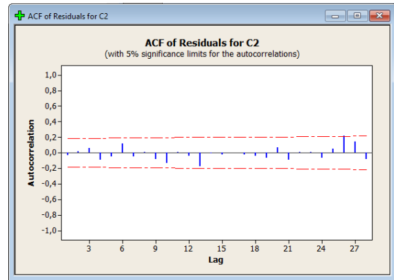
Gambar 7. Ploting Residual ACF Stasiun Kalijaran
